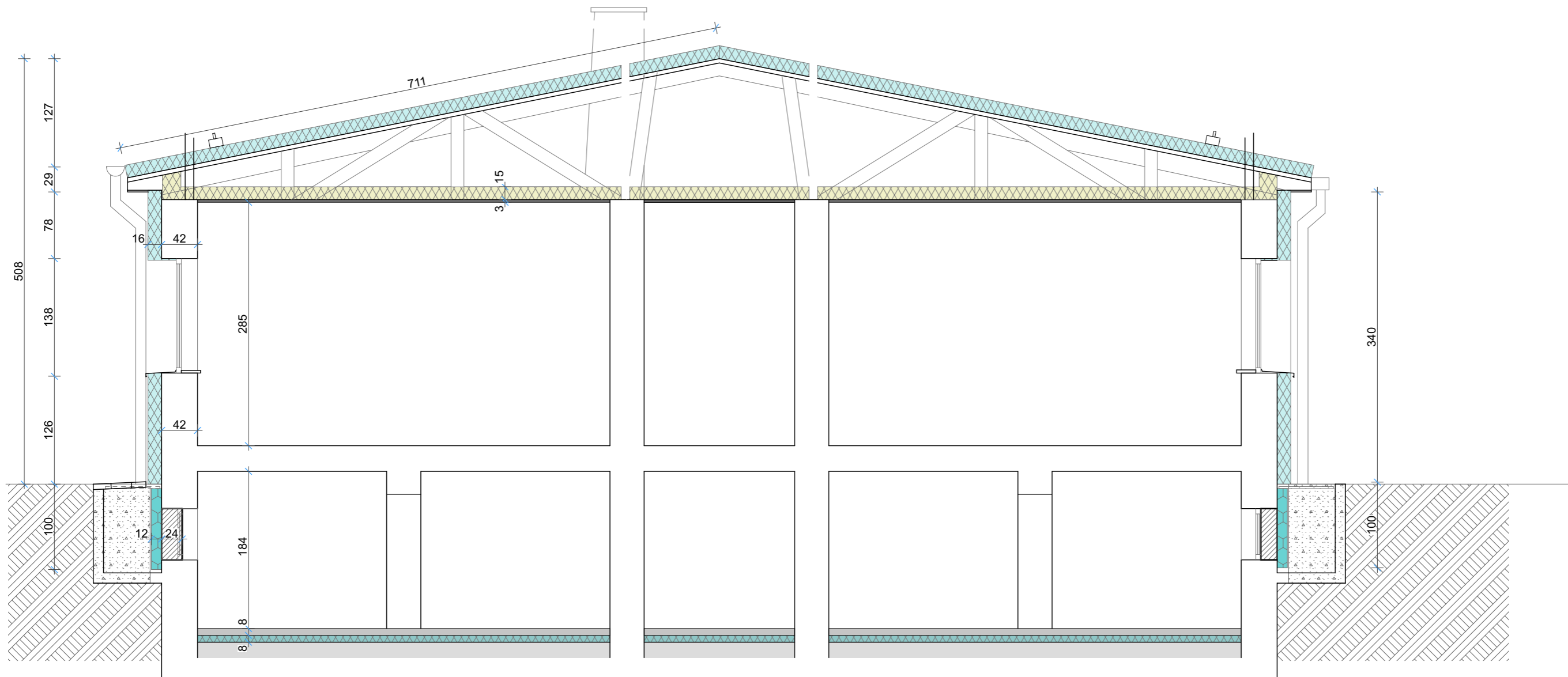
PRZEKRÓJ
