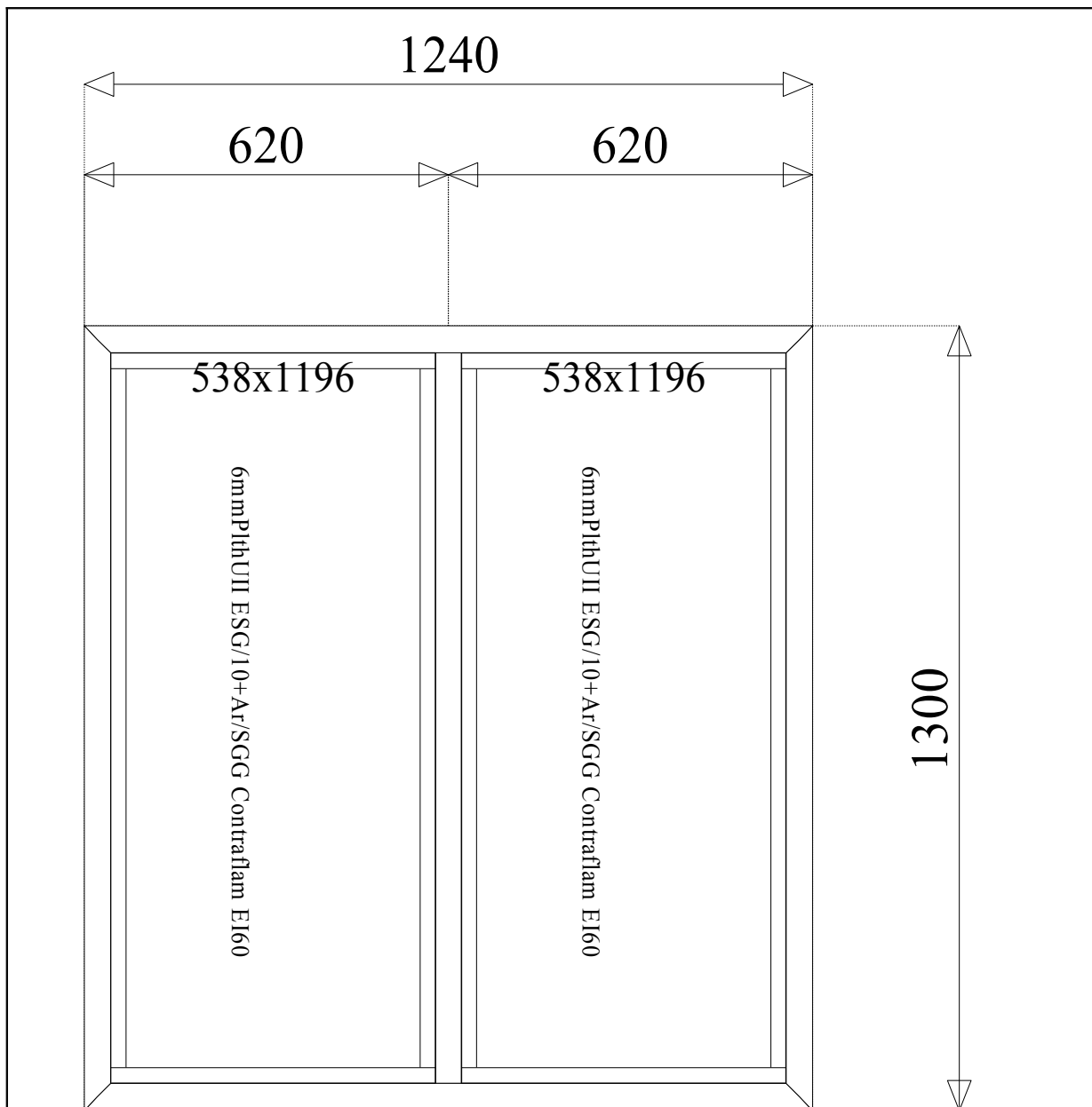
Widok konstrukcji od zewnątrz
