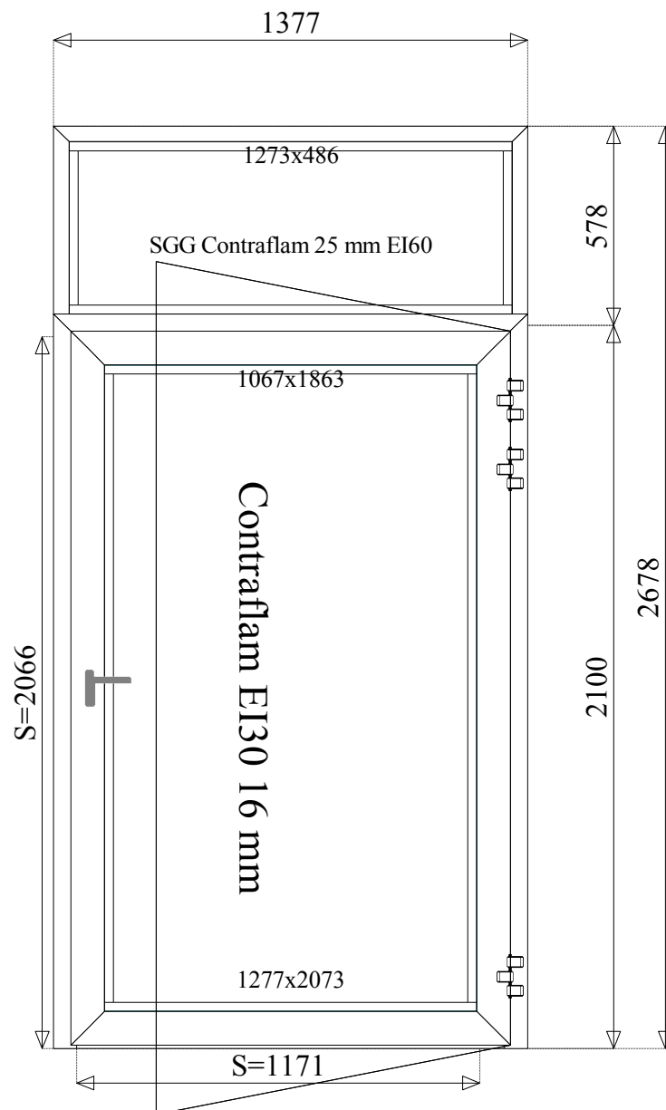
Widok konstrukcji od zewnątrz
