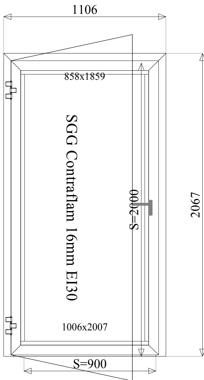
Widok konstrukcji od zewnątrz
