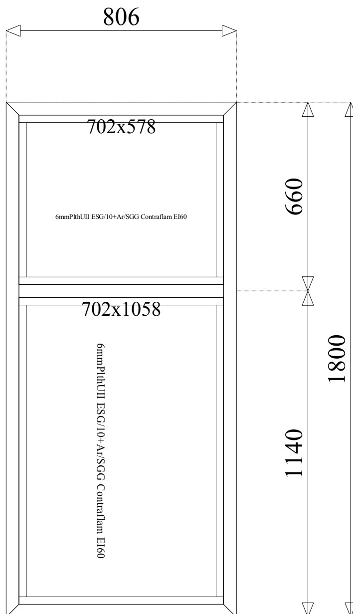
Widok konstrukcji od zewnątrz
