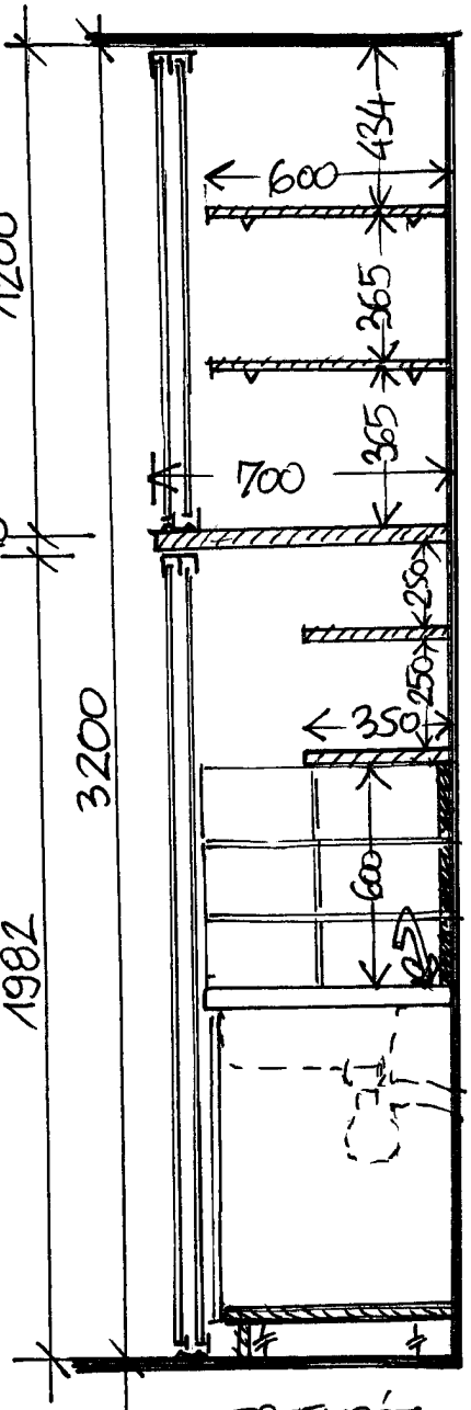
PRZEKRÓJ
