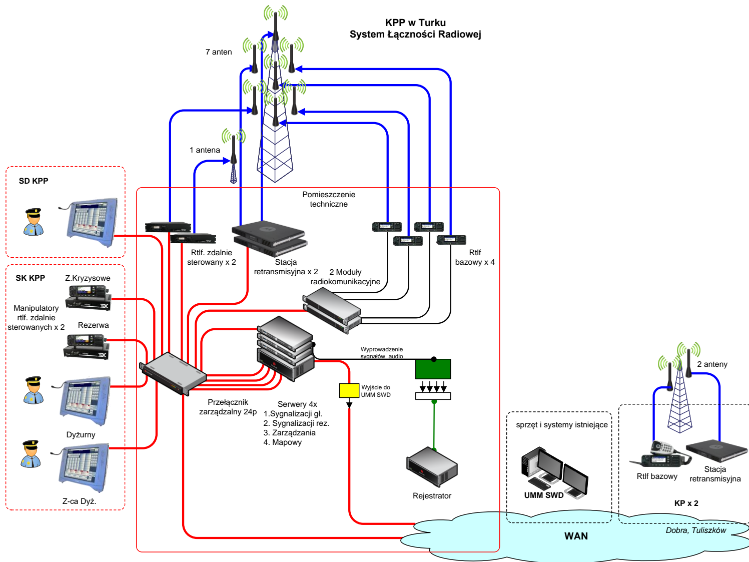
Rysunek 1 - Ogólny schemat systemu radiokomunikacyjnego dla KPP w Turku
